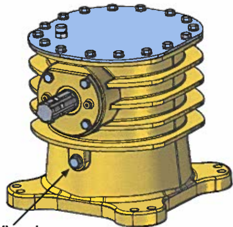
Tappo di scarico
