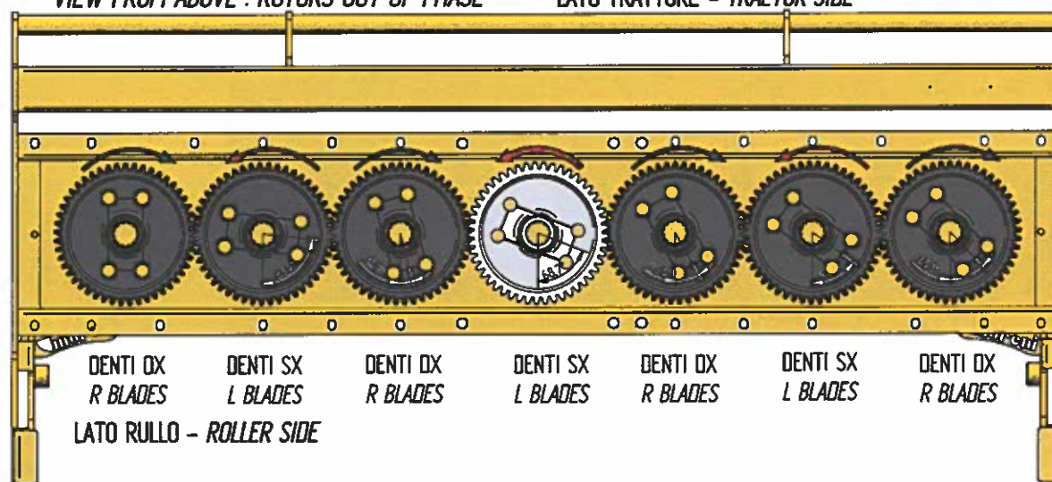
VISTA DALL'ALTO : ROTORI SFASATI VIEW FROM ABOVE : ROTORS OUT OF PHASE
