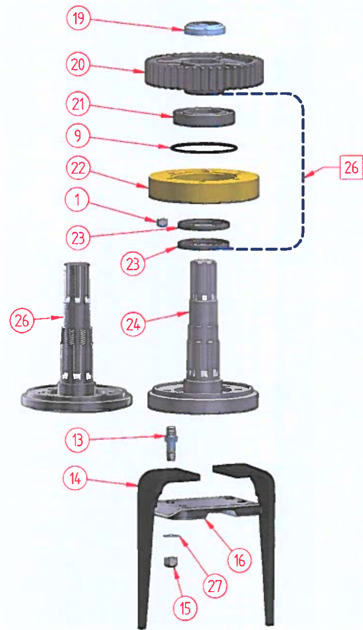
MOVIMENTAZIONE KRONOS - KRONOS ROTORS
