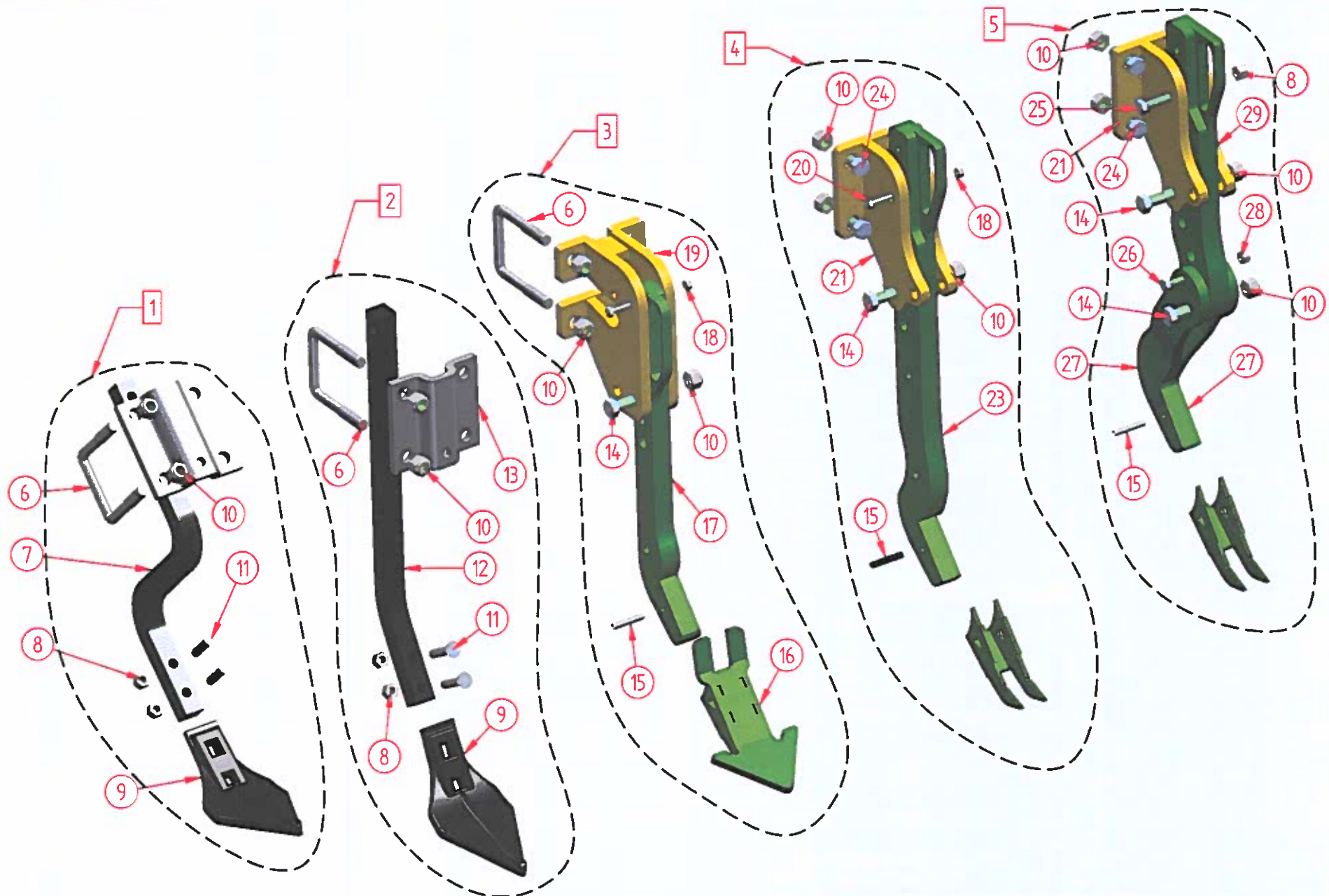
ROMPITRACCIA ERPICI - WHEEL MARK ERADICATOR
